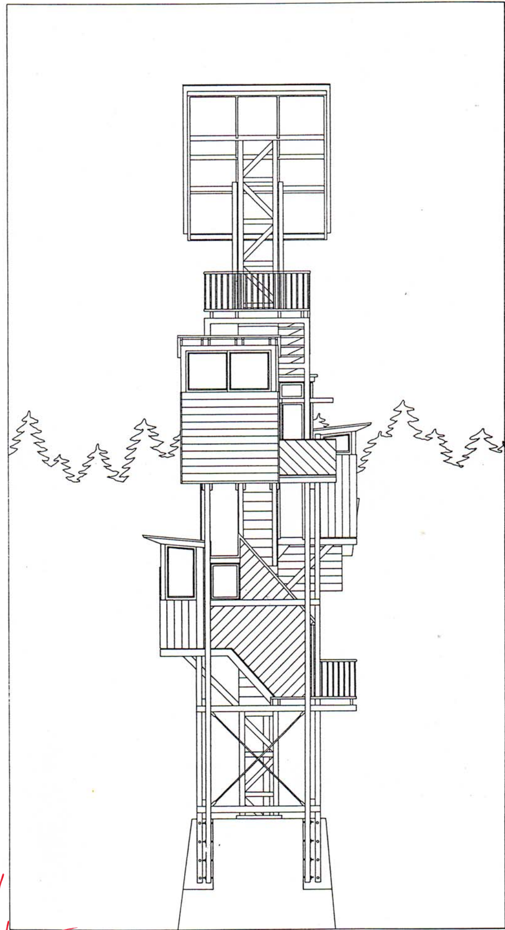
ANSICHT D
