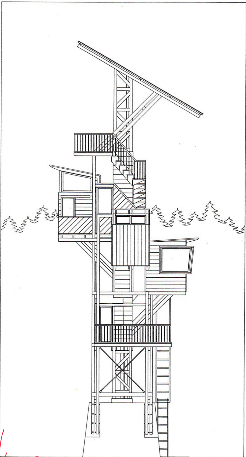
ANSICHT B
