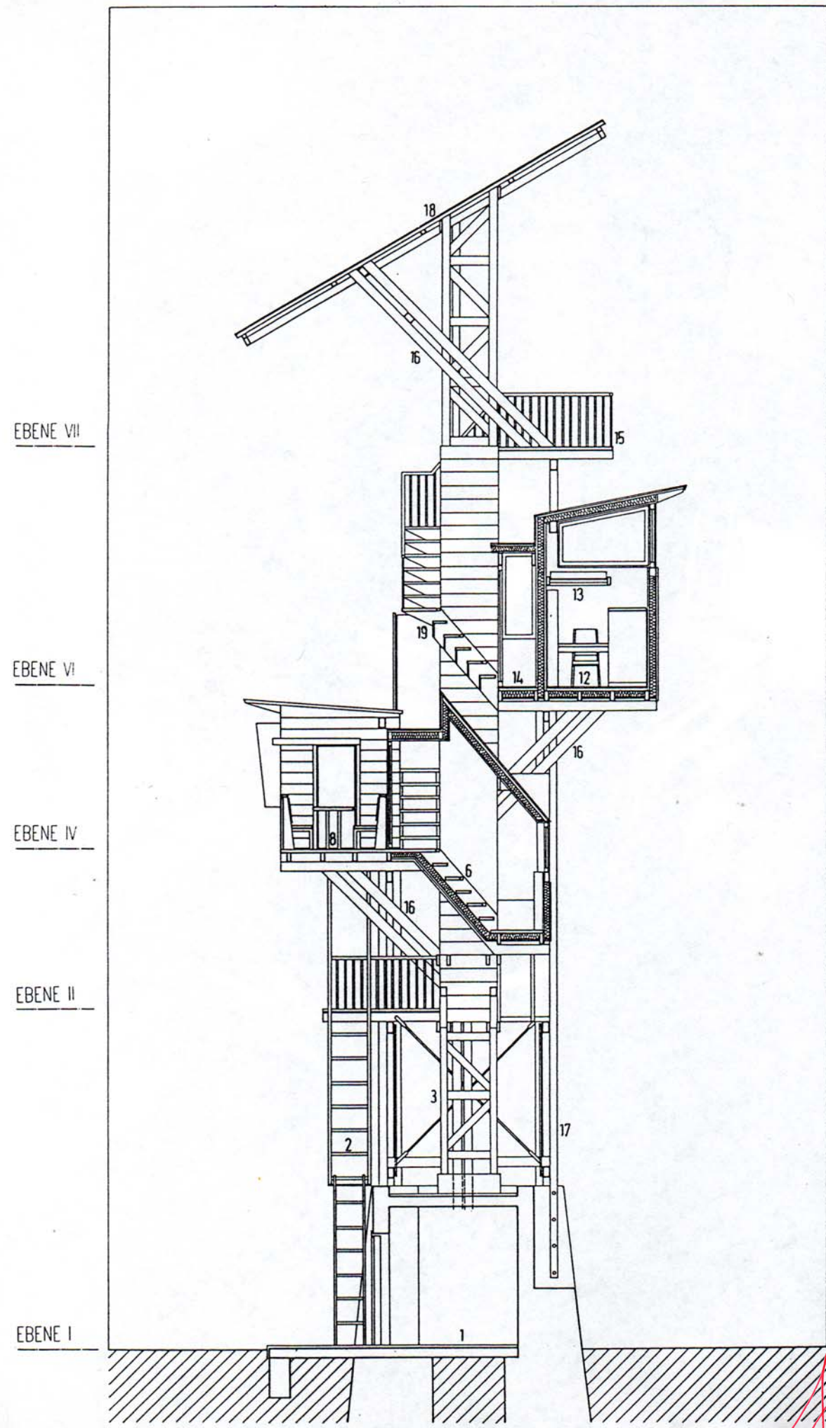
SCHNITT 1
