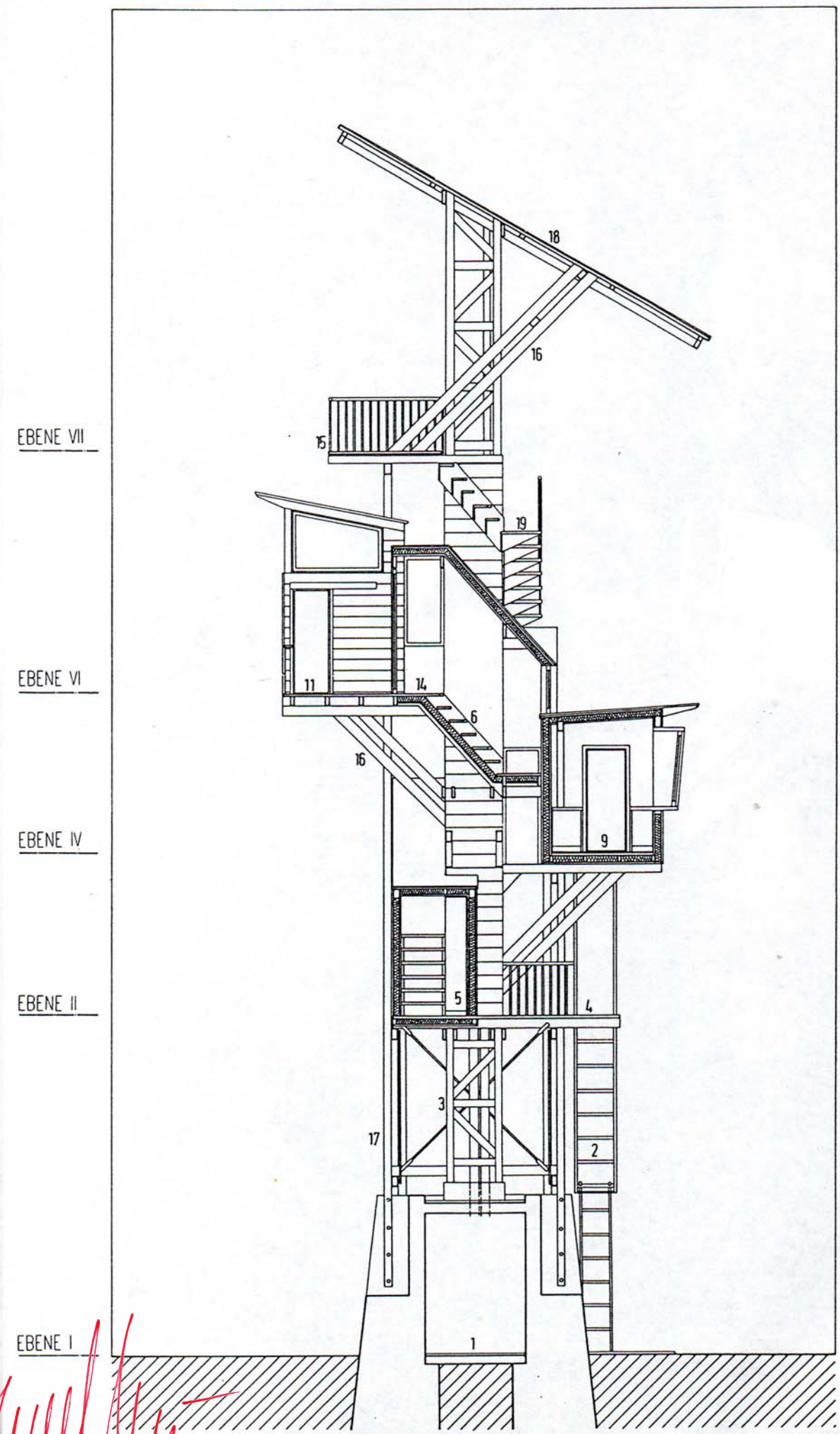
SCHNITT 2
